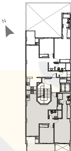
PLANTA 2°, 4° Y 6° PISO
