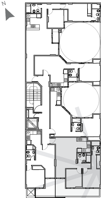
PLANTA 1º a 6º PISO
